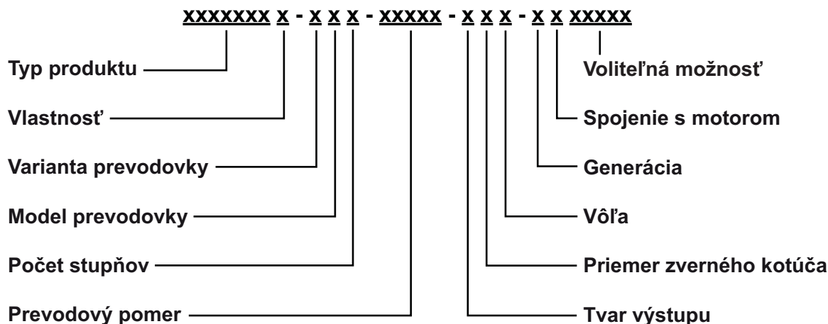
Tbl-5: Typový štítok (vzorové hodnoty)
